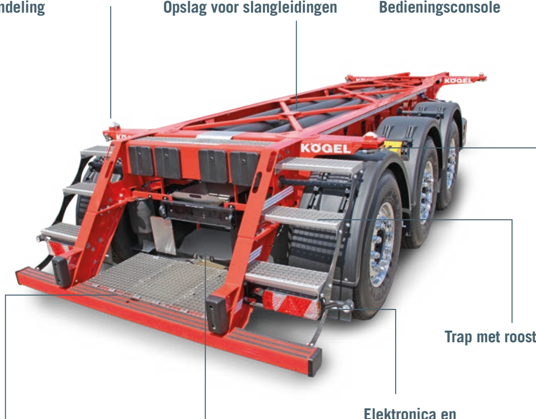
Werkplatform
